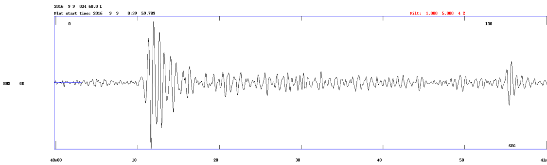
Signal på seismografen i Danmarkshavn, 9. september 2016:
