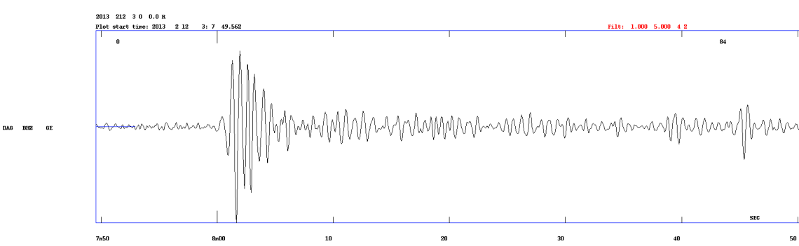
Signal på seismografen i Danmarkshavn, 12. februar 2013:
