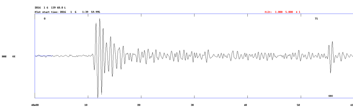
Signal på seismografen i Danmarkshavn, 6. januar 2016:
