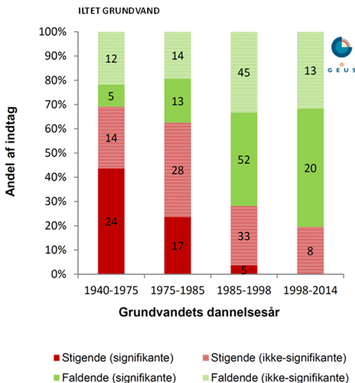
Figur 26. GRUMO. Iltet grundvand: nitrat-trends i 303 overvågningsindtag i iltet grundvand i 4 perioder baseret på grundvandets dannelsesår. Analysen inkluderer i alt 3.233 prøver fra 250 indtag, hvor tidsserierne dækker mindst 8 år. Tallene inden i søjlerne angiver antallet af indtag. Der er vist både signifikante og ikke-signifikante nitrat-trends på 95 % konfidensniveau. Figuren er baseret på data indsamlet fra 1988-2014.
