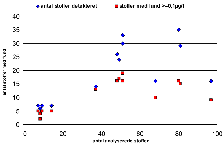
Figur 1 G. Antallet af fundne pesticider og metabolitter mod analyseprogrammets størrelse. Figuren er sammensat ud fra data fra tabel 1, og stoffer som kun er detekteret få gange er medtaget.
