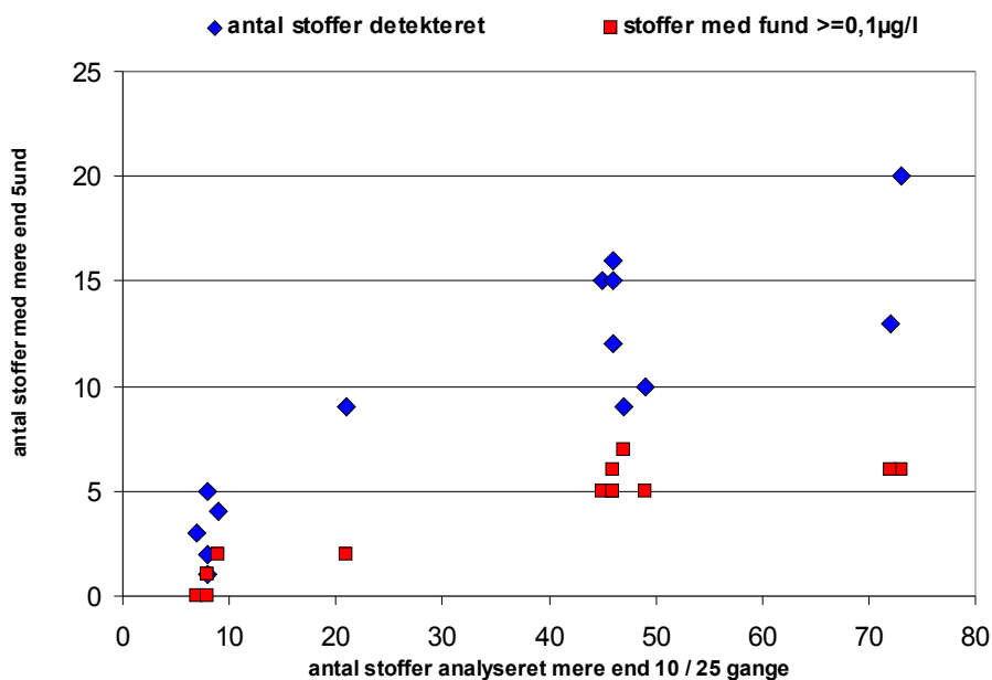
Figur 1 G. Antallet af fundne pesticider og metabolitter mod analyseprogrammets størrelse. Figuren er sammensat ud fra data fra tabel 1, og stoffer som kun er detekteret få gange er medtaget.
